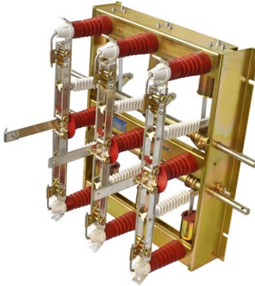
Figura 4. Seccionador tripolar de uso interior
