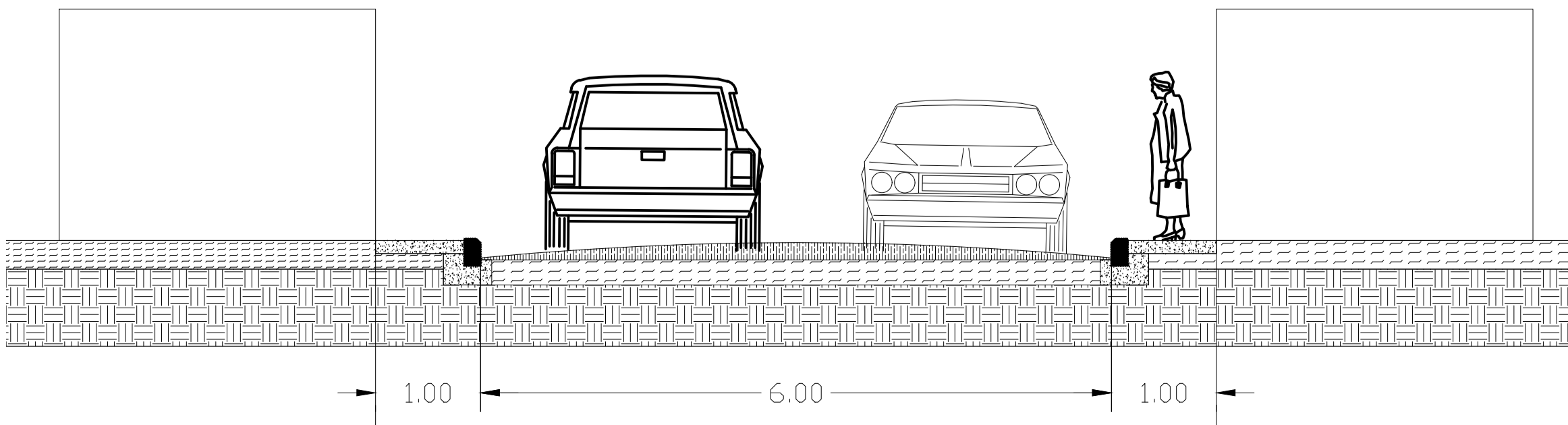
CALLE 28 A PERFIL ACTUAL ESCALA 1/50
