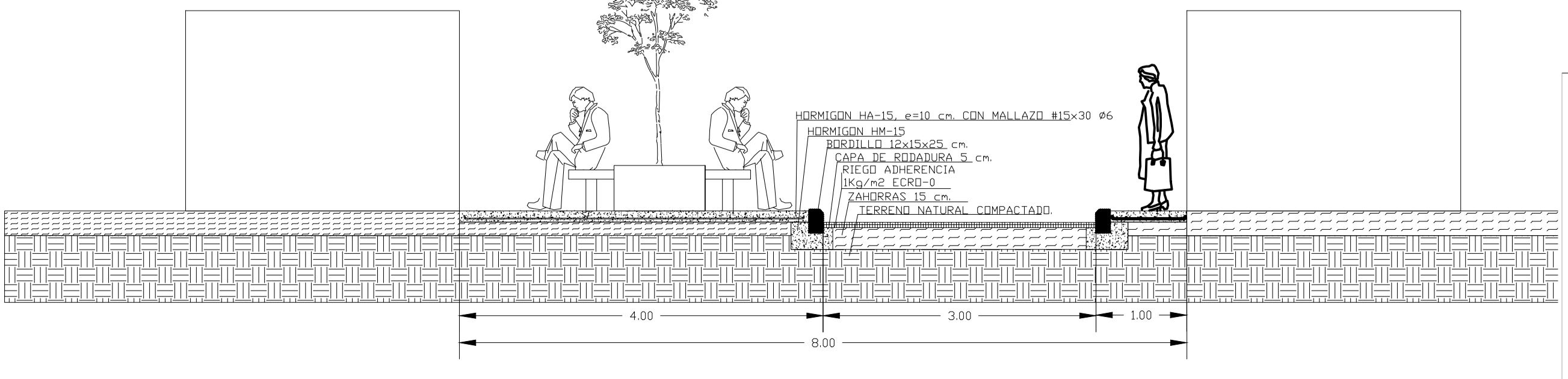
CALLE 28 A PERFIL PROPUESTO ESCALA 1/50
