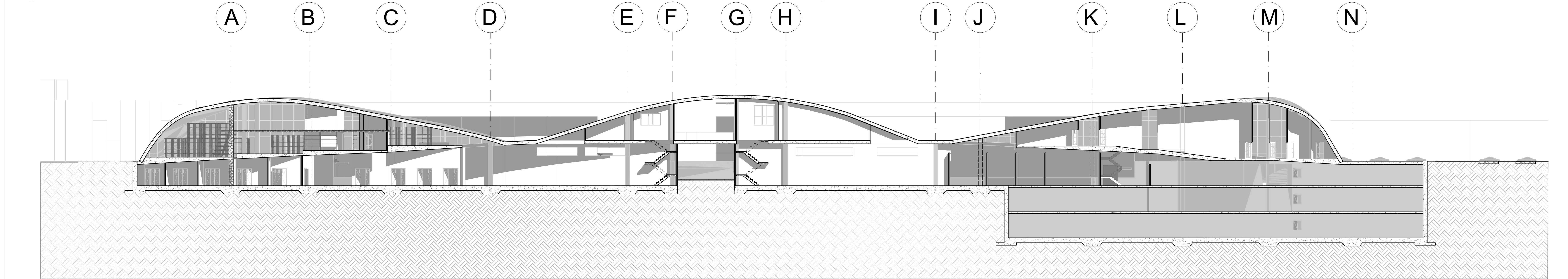
Sección longitudinal B-B' ESC. 1-200
