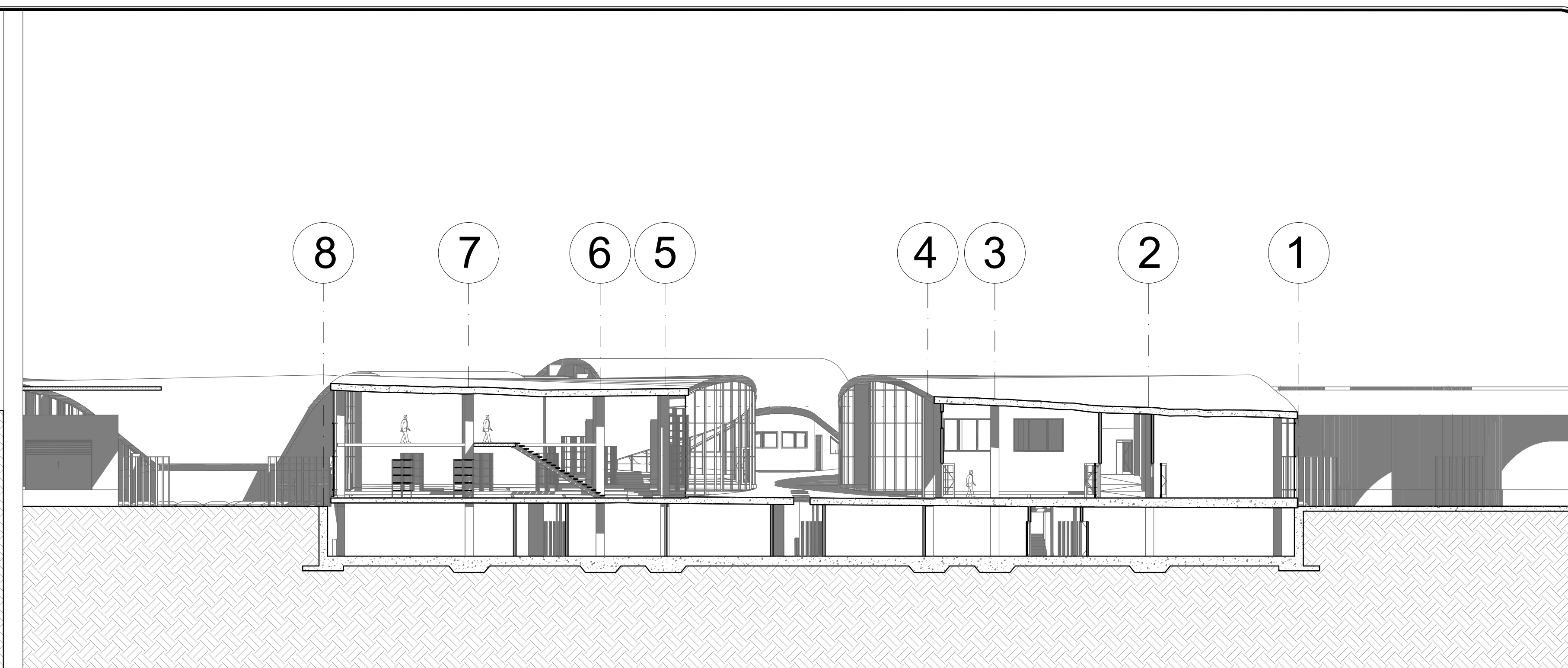
Sección transversal D-D' ESC. 1-200
