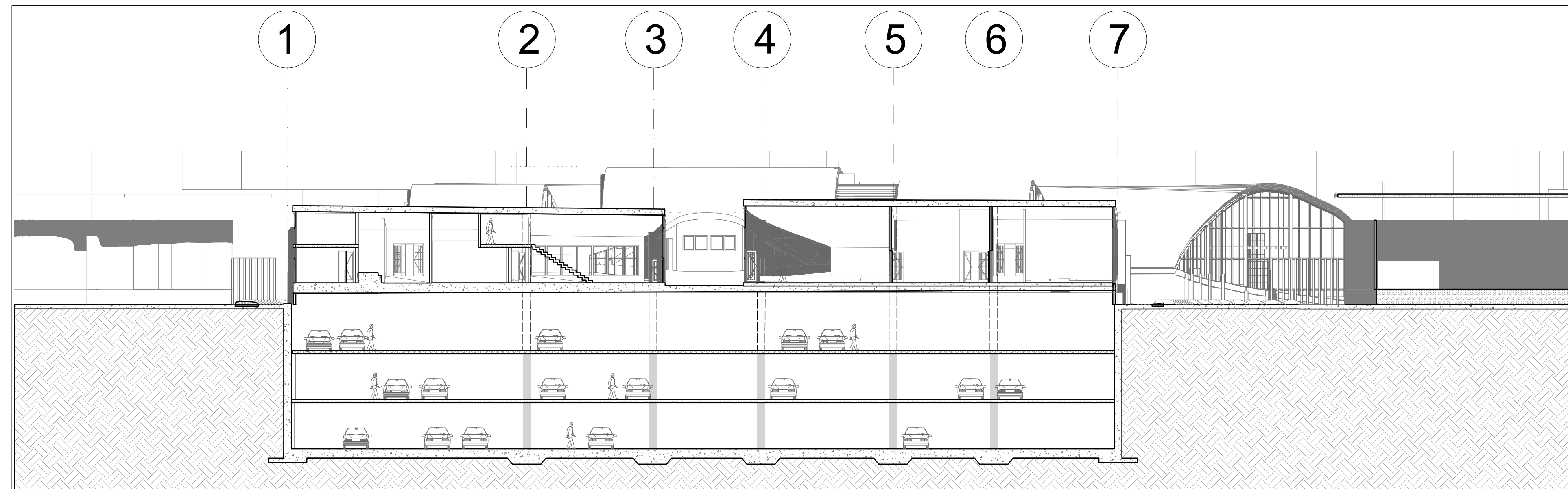
Sección transversal E-E' ESC. 1-200
