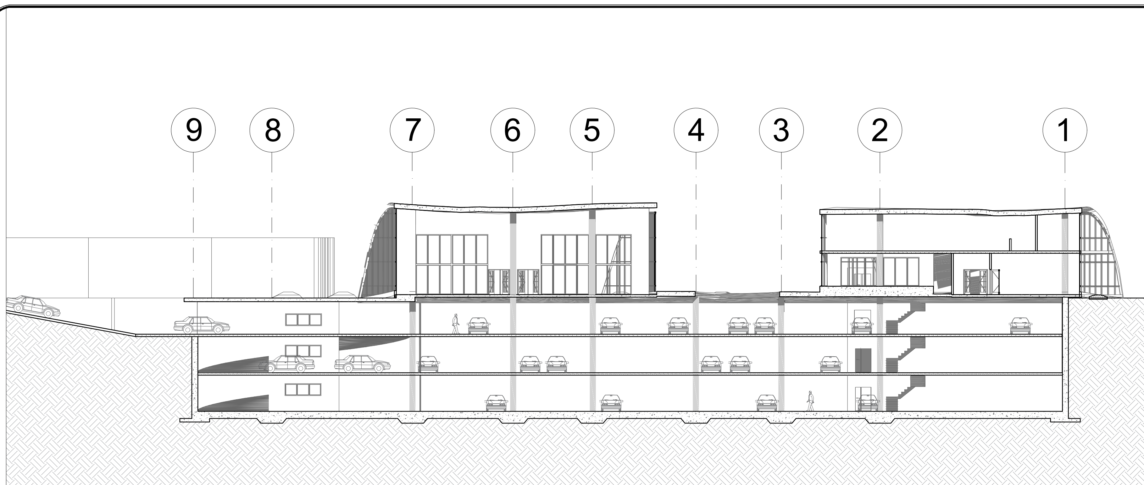
Sección transversal C-C' ESC. 1-200
