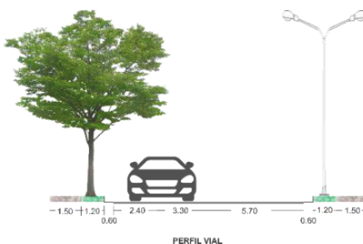
Ilustración 19: Perfil vial V2 Espinal
