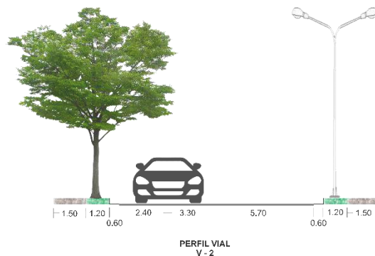
Ilustración 22. Vía y perfil vial Espinal - Caimanera
