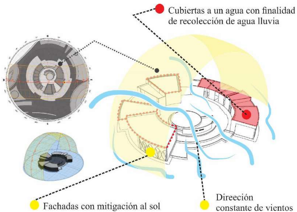
Ilustración 30. Esquema bioclimático del proyecto.
