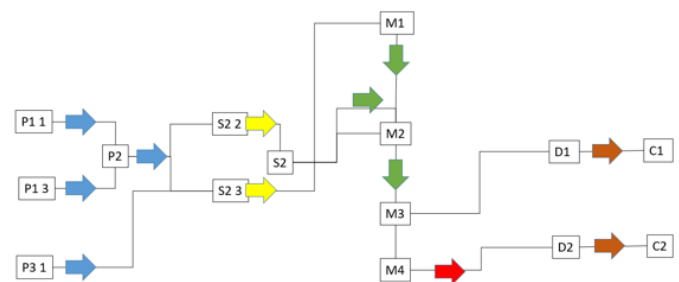
FIGURA 7 Propuesta de diagrama de hilos en la provincia de Lengupá.
