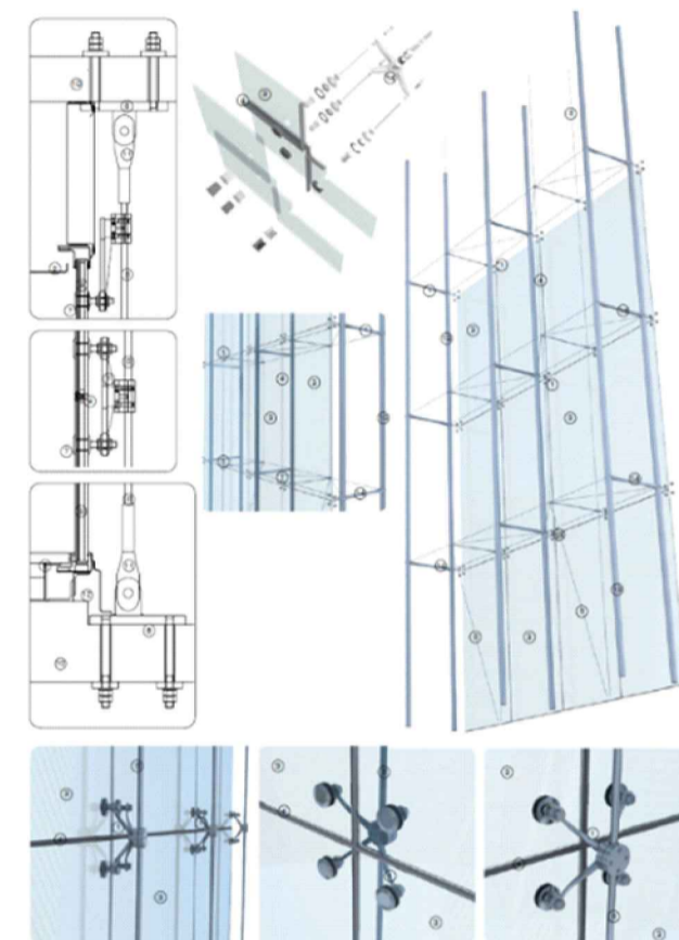
DETALLLE VIDRIOS
