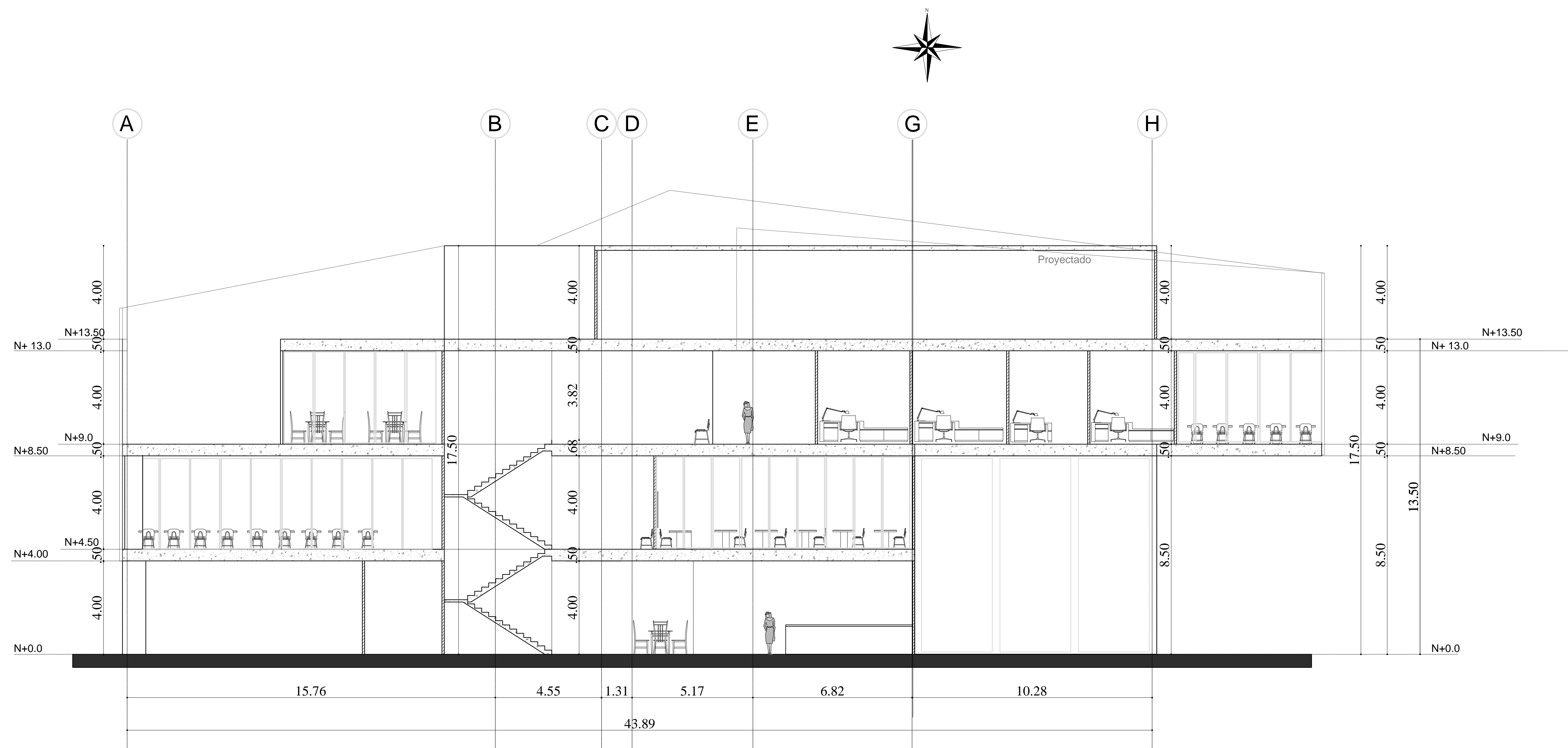
CORTE TRANSVERSAL
