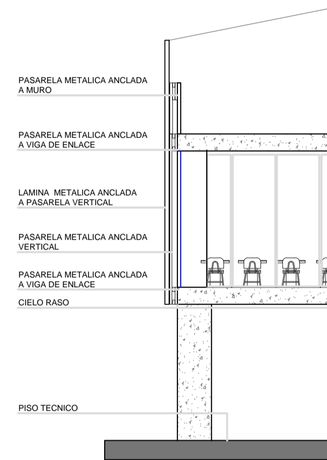
DETALLE FACHADA
