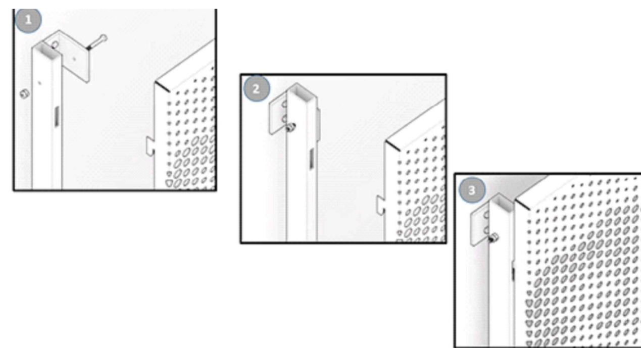
DETALLE ANCLAJES ENVOLVENTES
