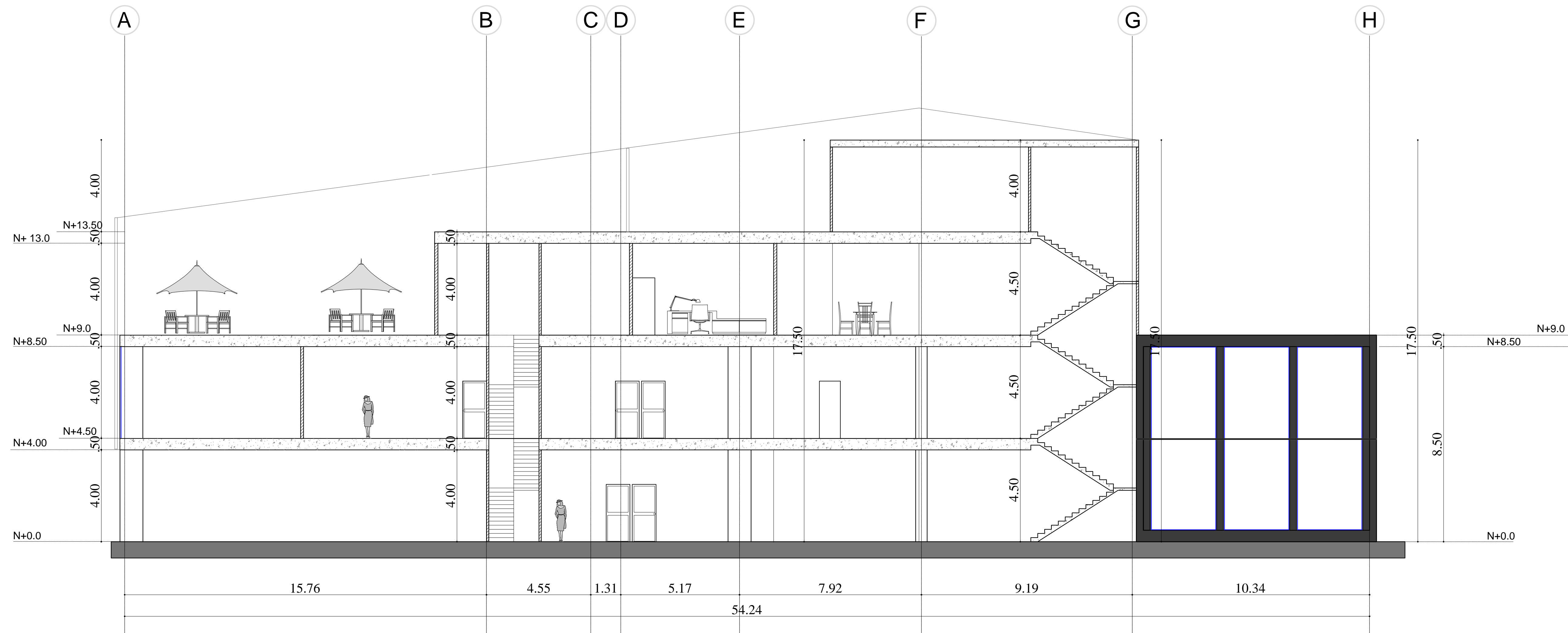
CORTE LONGITUDINAL
