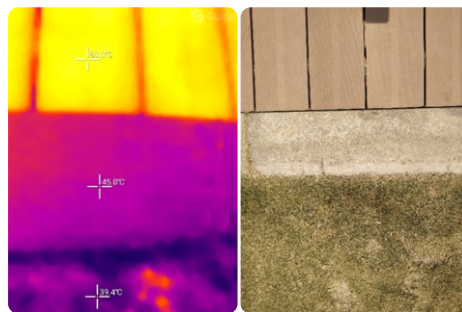
Relación del comportamiento térmico del material Deck, cemento y prado (Diferencia de 15°C).
