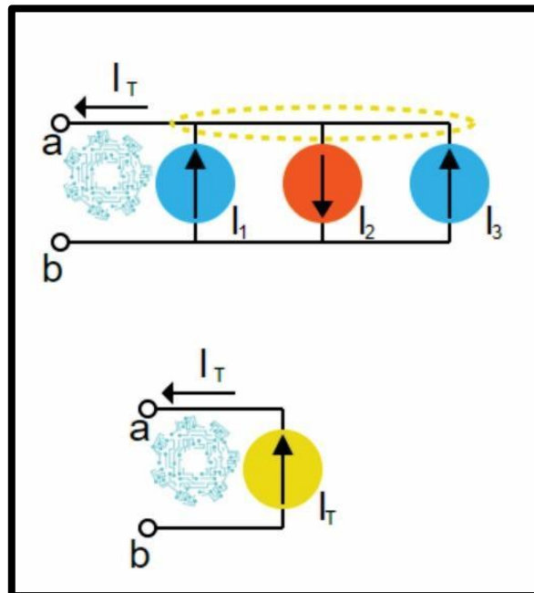
Figura 6 Ley Kirchhoff en paralelo
