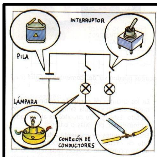
Figura 1 Ejemplo Circuito Eléctrico Básico
