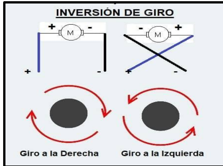
Figura 8 Ejemplo inversor de giro
