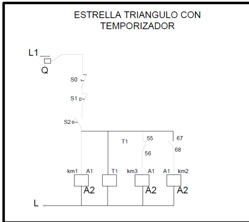
Figura 15 Diagrama unifilar estrella triangulo con temporizador
