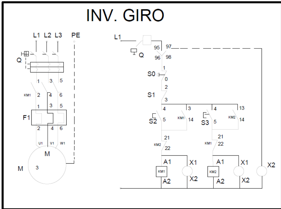
Figura 14 Diagrama Unifilar Inversión de giro
