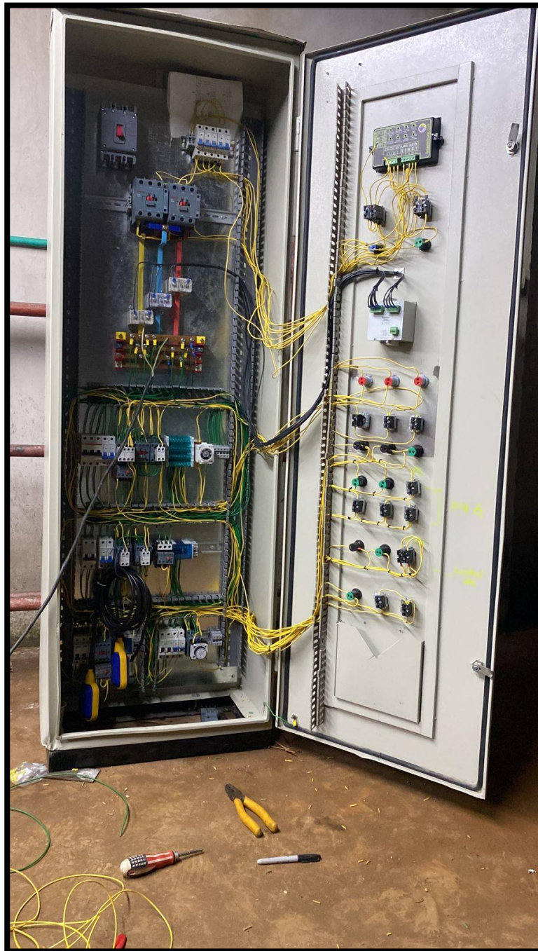
Figura 31 Construcción de tablero eléctrico didáctico
