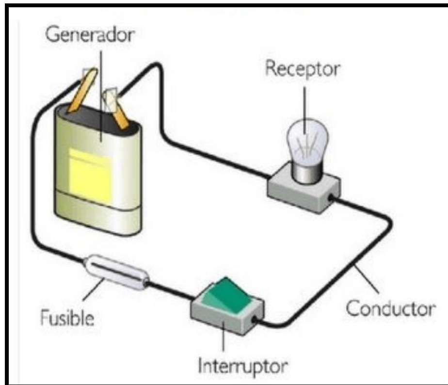
Figura 3 Esquema de cortocircuito
