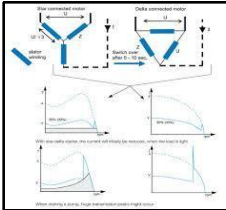
Figura 7 Diagrama arranque estrella triangulo
