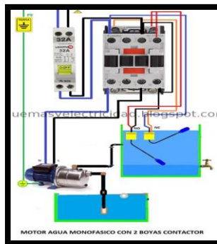
Figura 9 Sistema control de nivel por medio de flotadores
