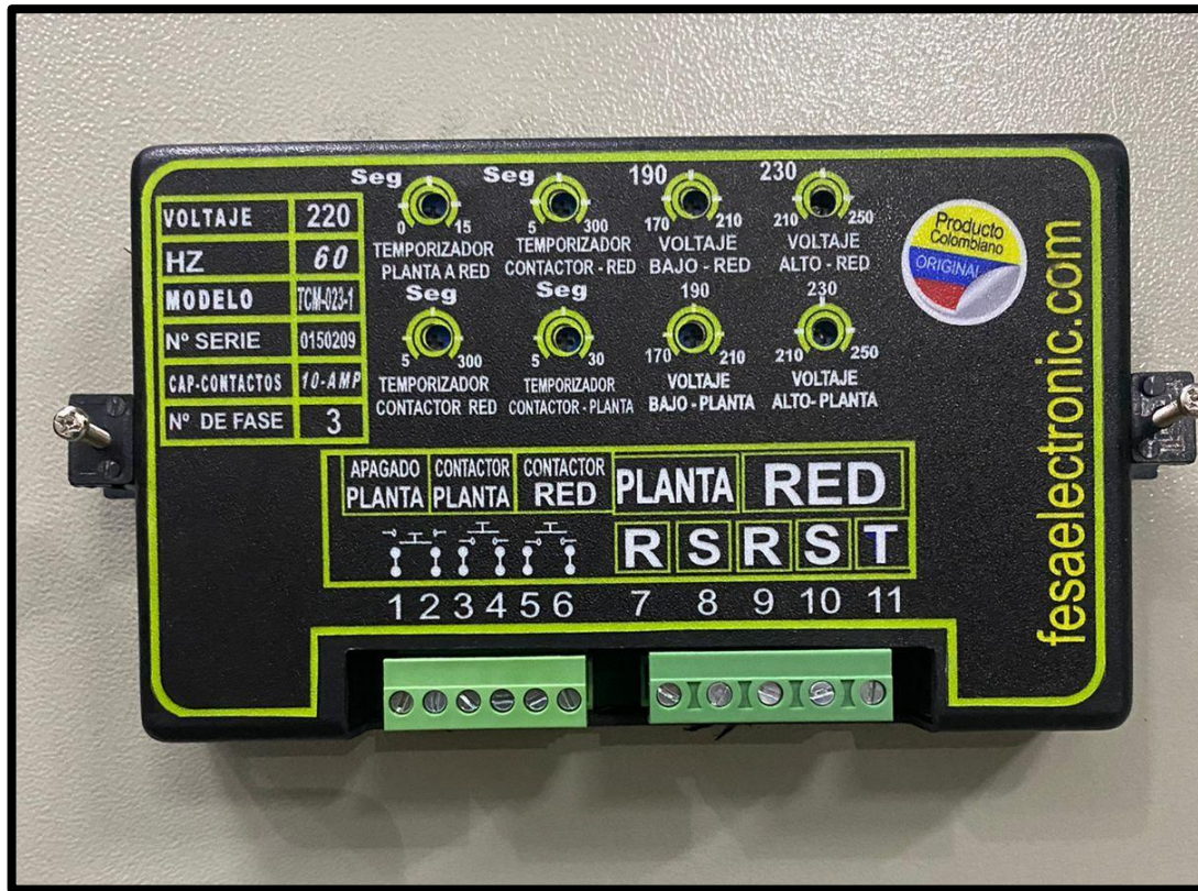
Figura 24 Instalación módulo de transferencia
