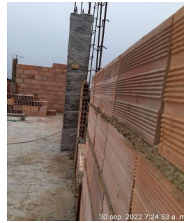
Descripción: armado de columnetas
