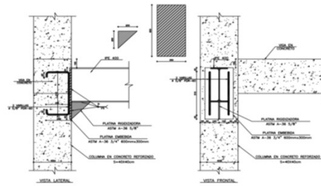
Descripción: detalle de instalacion de platina
