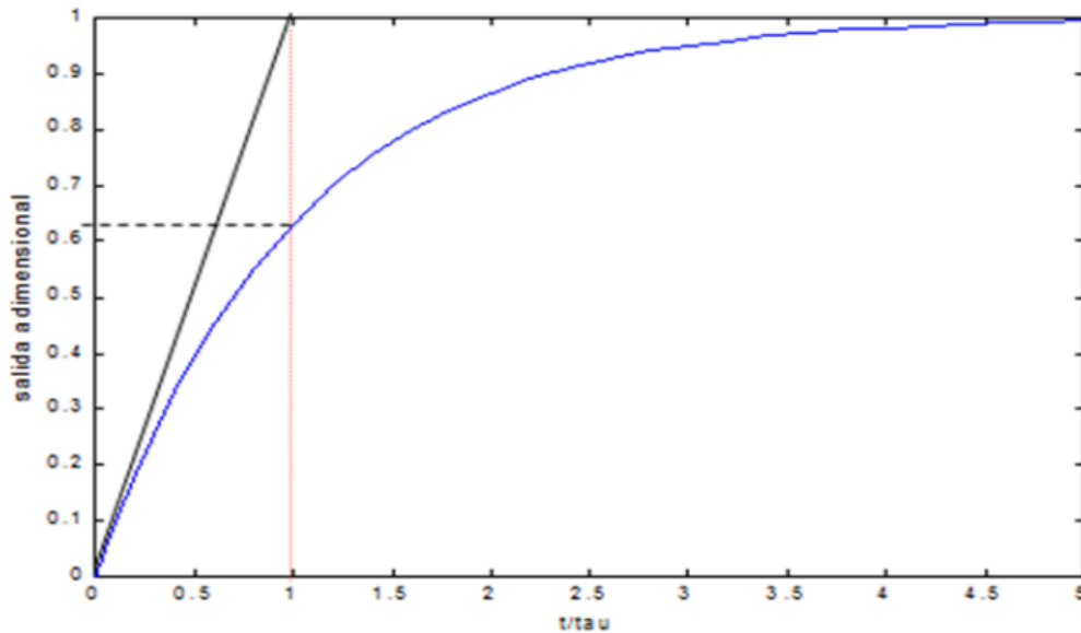
Figura 5-2: Respuesta de la Función de Tránsito del Panel Fotovoltaico.
