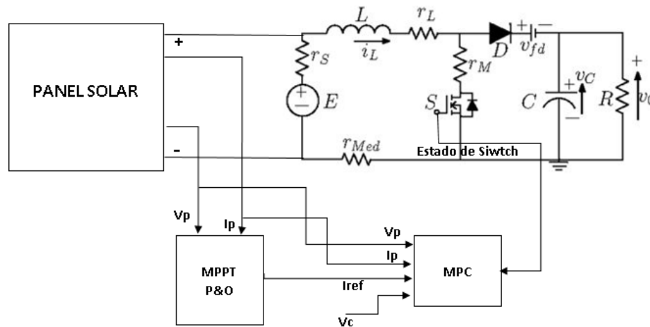
Figura 6-7: Esquema de MPC para MPPT
