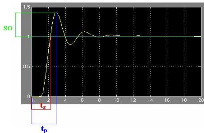
Figura 5-5: Respuesta al Paso de la Función de Transferencia.
