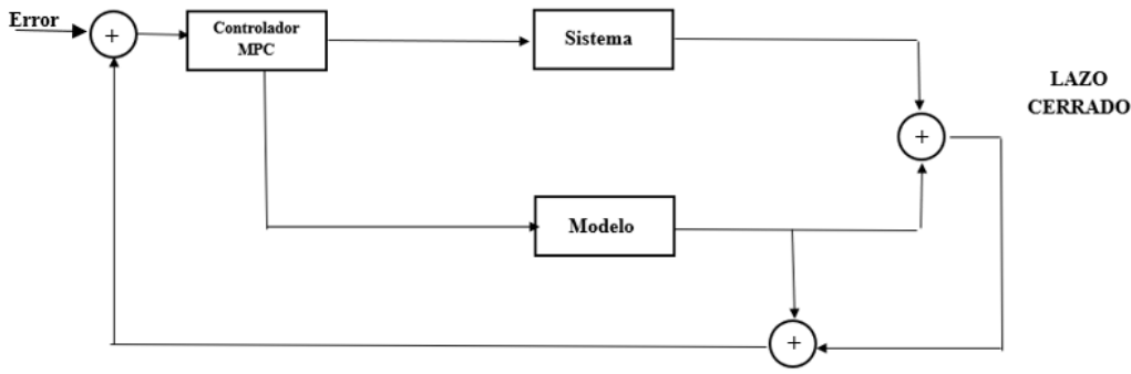
Figura 6-5: Error Para el Muestreo en Lazo Cerrado del MPC
