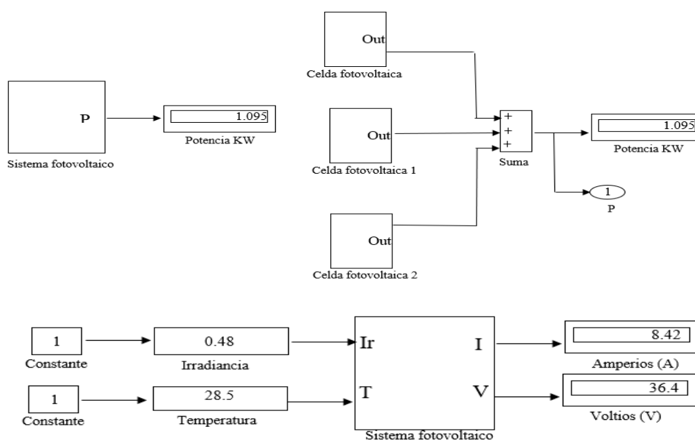
Figura 4-9: Simulación del Panel Fotovoltaico en Simulink.
