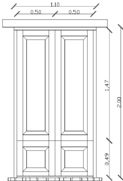
Alzado ventana principal
