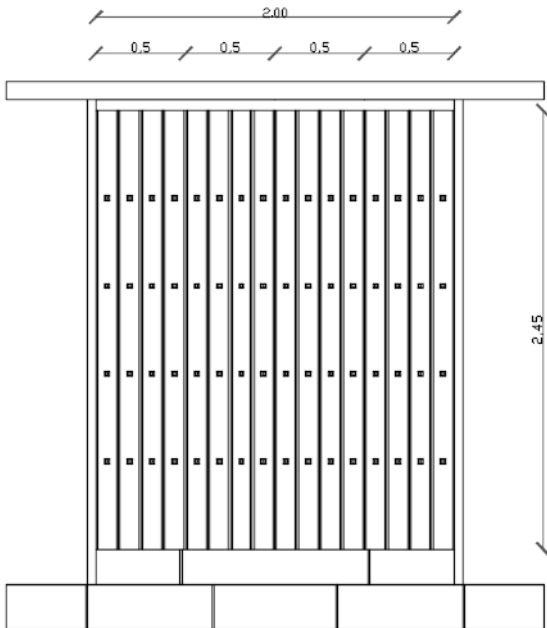
Alzado puerta principal
