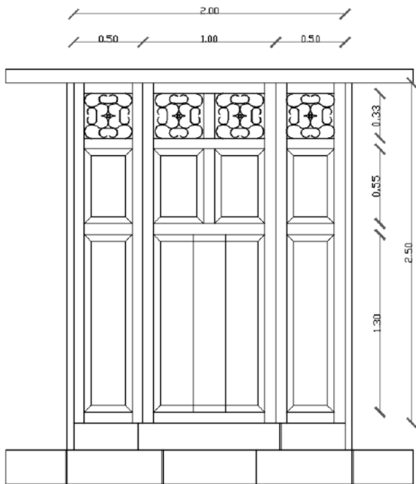
Alzado puerta principal
