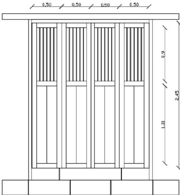
Alzado puerta principal
