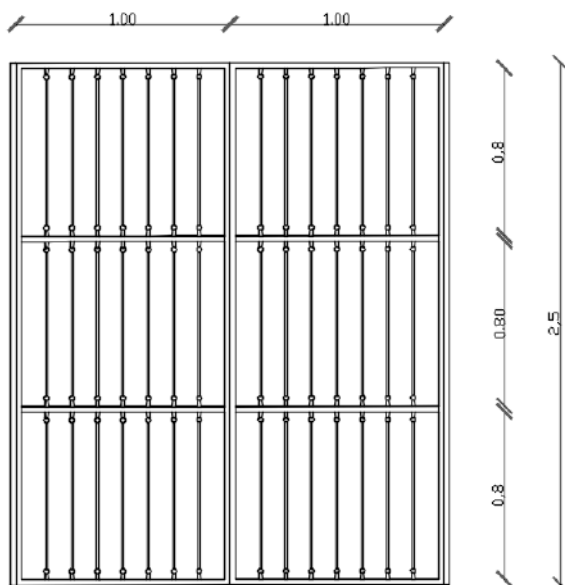
Alzado Reja
