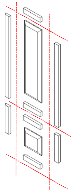
Explotado
