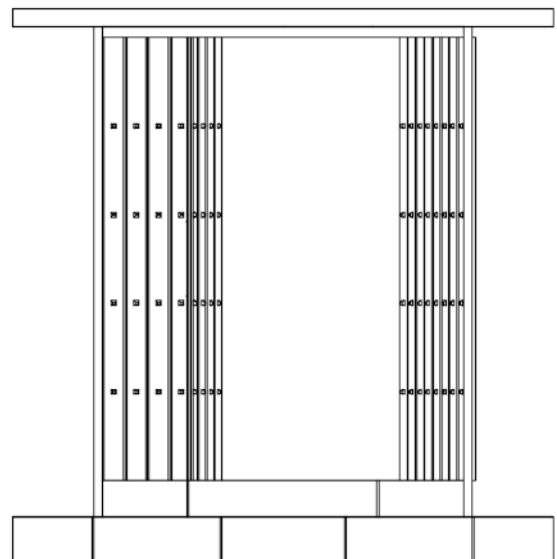
Alzado puerta principal abierta en el centro lateral
