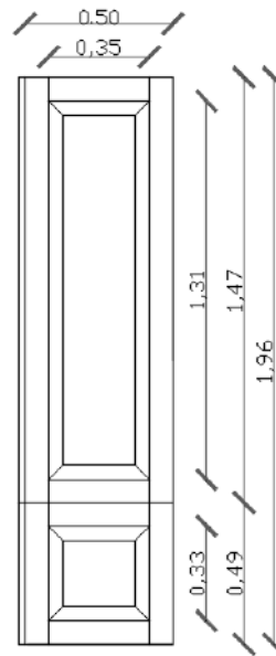
Alzado hoja puerta
