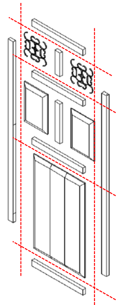
Explotado
