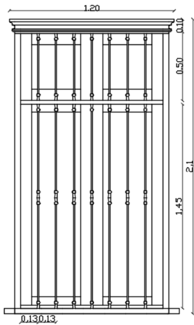
Alzado Ventana
