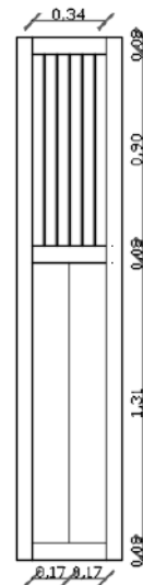
Alzado hoja puerta
