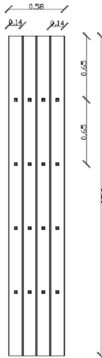
Alzado hoja puerta
