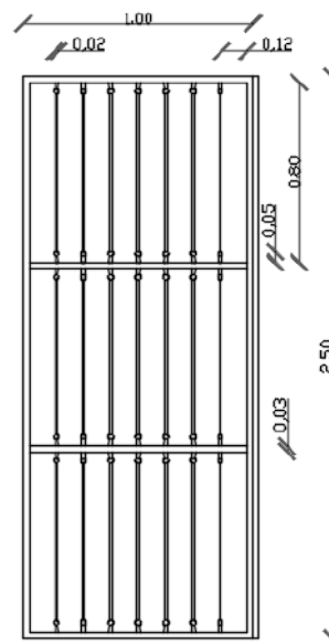
Alzado hoja reja
