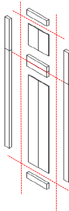
Explotado
