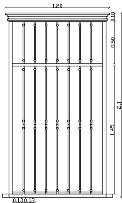
Alzado Reja
